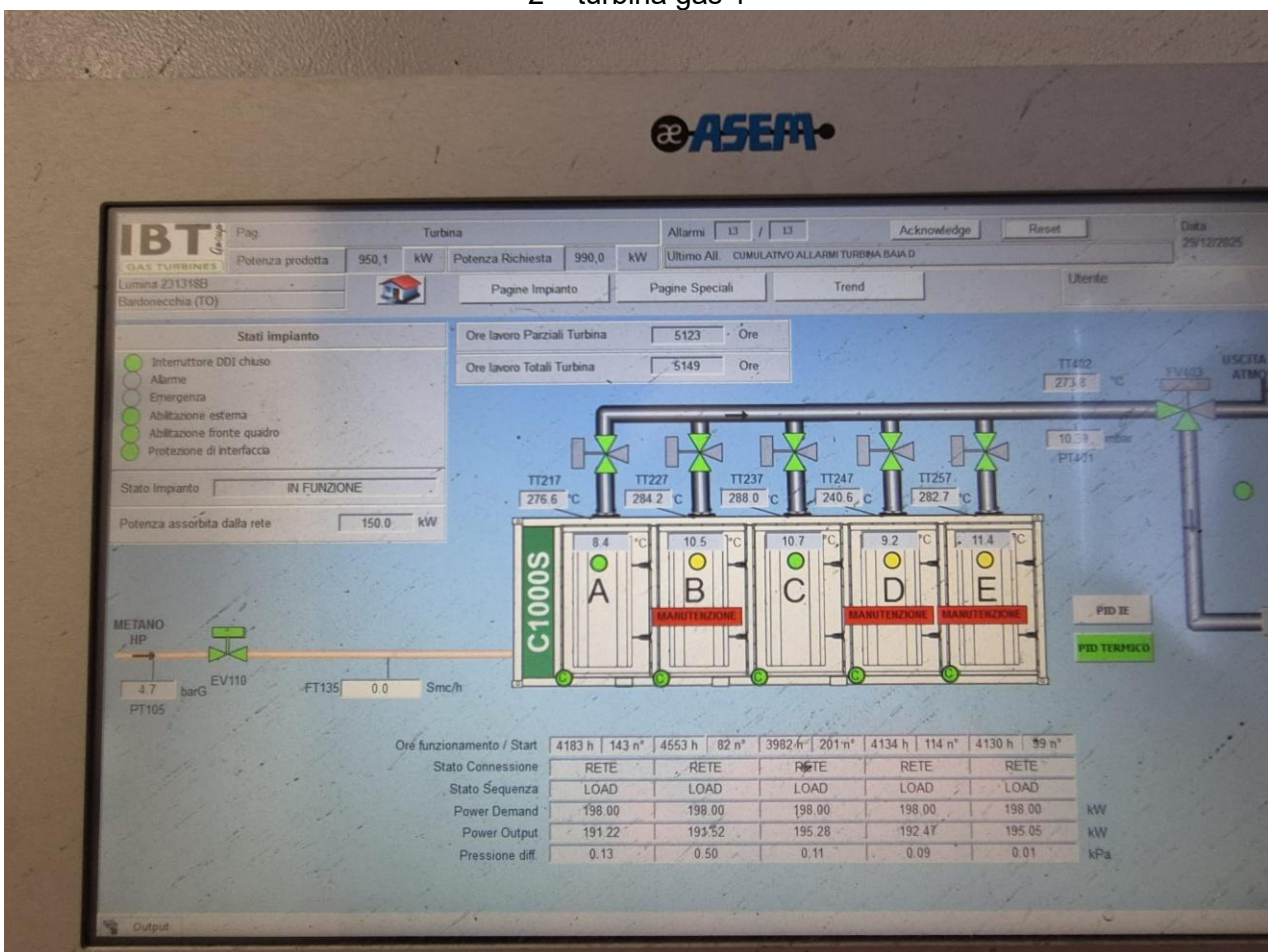
3 – quadro sinottico turbina gas
