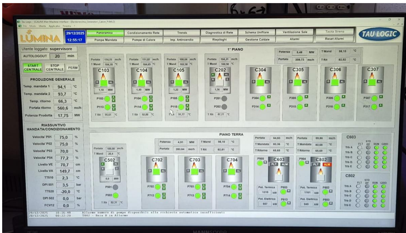
1 – quadro sinottico generatori terminale centrale controllo
